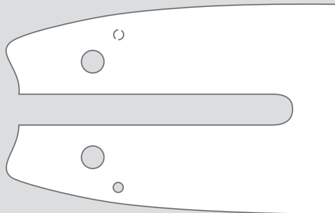
AANSLUITING: A074 Stihl en anderen 3/8" hobby 1,1 met 1,3 mm
