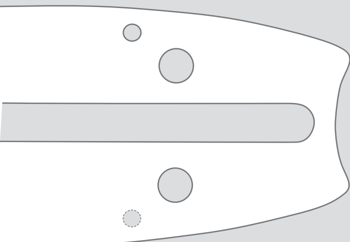
AANSLUITING: D009 Dolmar, Husqvarna, Solo 3/8" 1,5 mm
