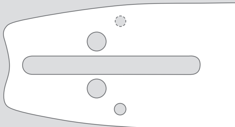
AANSLUITING: A095, K095 Dolmar, Husqvarna, Solo en anderen 325" 1,3 mm met 1,5 mm 3/8" 1,5 mm
